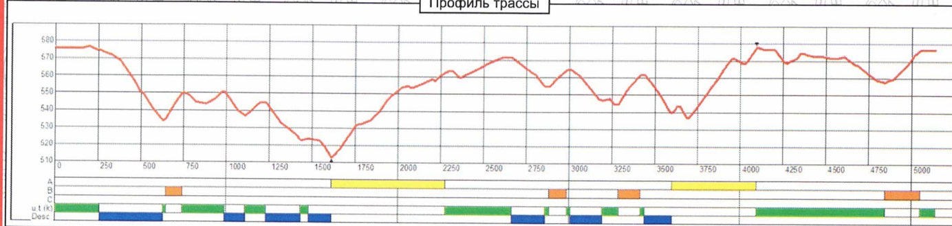
Профиль трассы
