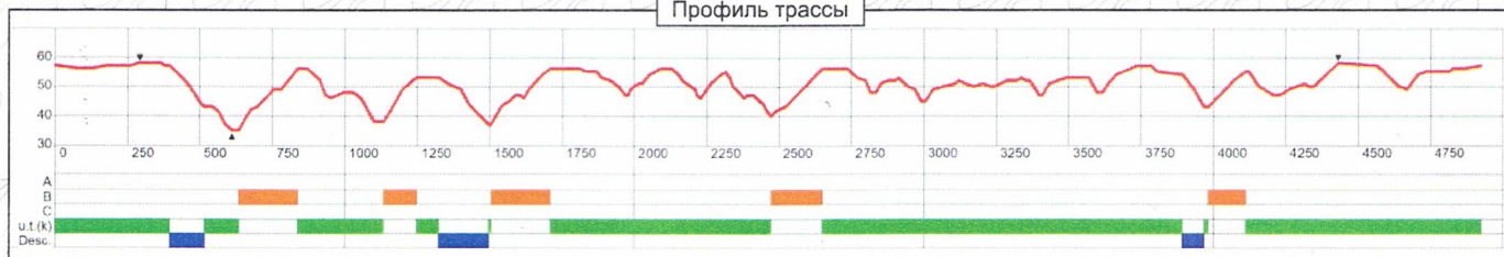
Профиль трассы
